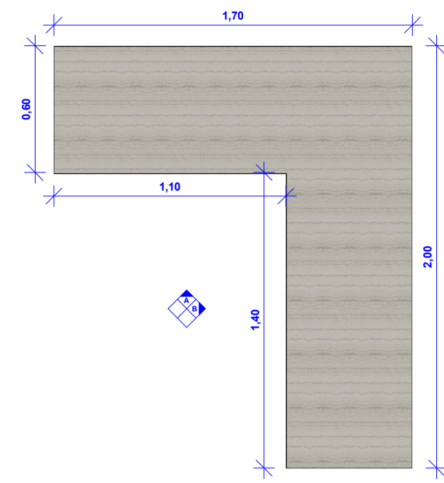
4 PLANTA DA MESA 1
